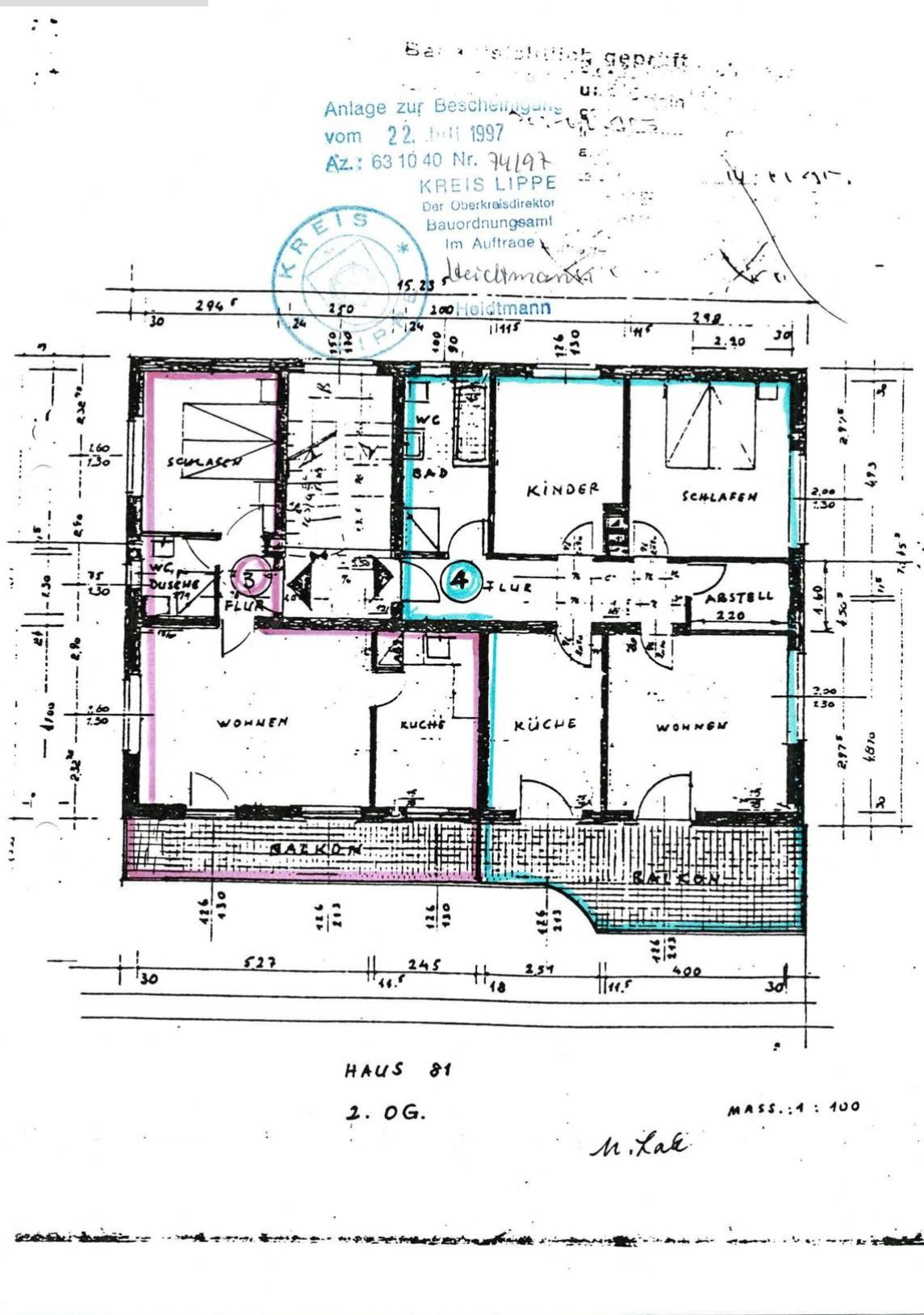
Grundriss 2 OG_Brunnenstraße 81-1
